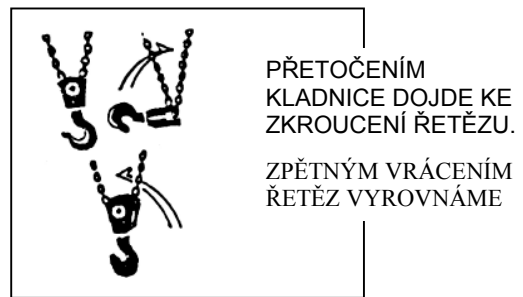
Obr. 6.2b Přetočení kladnice
