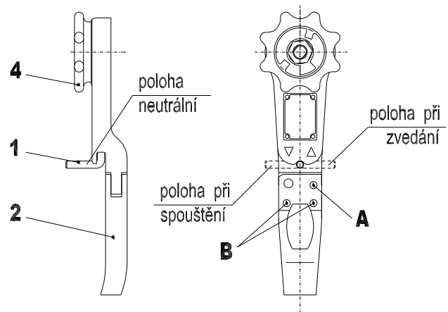
Obr. 6.3 – Nastavení délky řetězu
